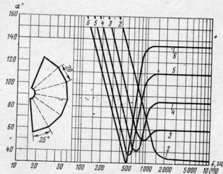
Рис. 82. Угловая ширина диаграммы направленности секционированного рупора: \alpha — угловая ширина основной части диаграммы; 2, 3, 4, 5, 6 — число ячеек
