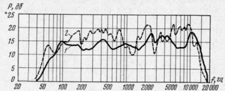
Рис. 44. Частотные характеристики громкоговорителей: 1 — 30А-46; 2 — 30А-68
