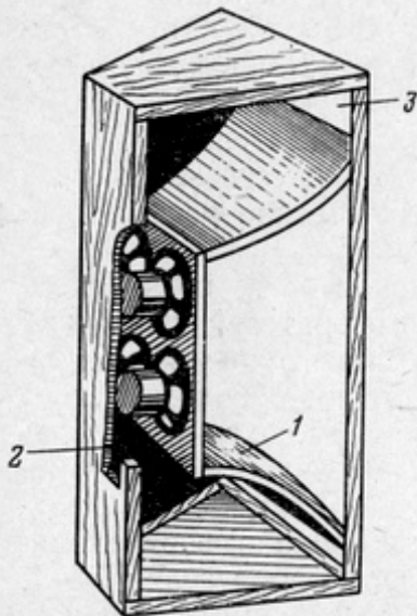
Рис. 80. Схема акустического оформления низкочастотного громкоговорителя:
