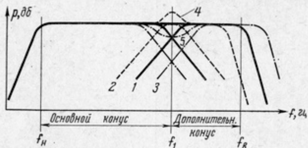
Рис. 39. Схема согласования характеристик основного и дополнительного конусов:
