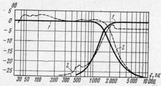
Рис. 77. Частотные характеристики разделительного фильтра двухполосного громкоговорителя: 1 — на активной нагрузке; 2 — на реальной нагрузке (головки)
