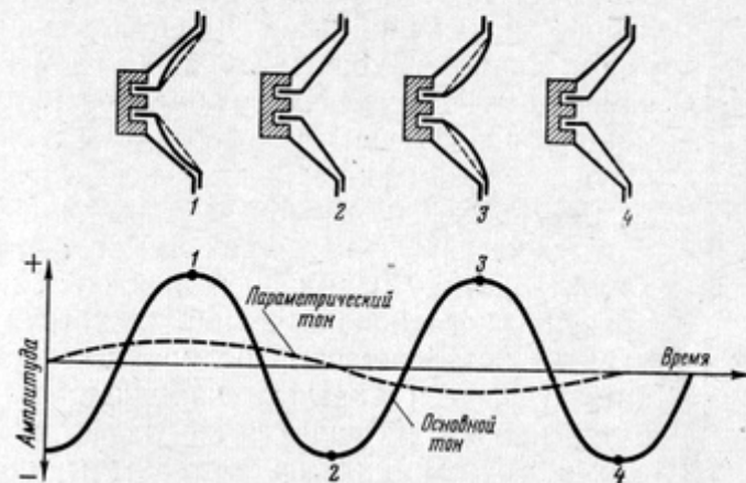
Рис. 51. Параметрические колебания диффузора с прямолинейной образующей
