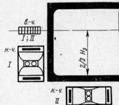
Рис. 115. Неправильное размещение звеньев двухполосного громкоговорителя
