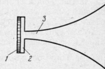
Рис. 58. Схема рупорного громкоговорителя:
