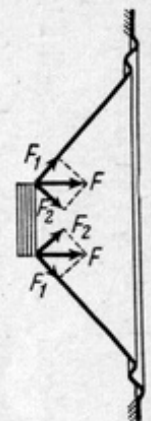
Рис. 47. Разложение на составляющие силы, приложенной к диффузору
