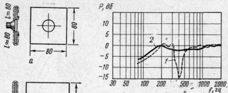
Рис. 24. Зависимость частотной характеристики от формы экрана: 1 — квадратный (0,8 × 0,8 м), отверстие в центре; 2 — прямоугольный (1,0 × 2,0), отверстие смещено от центра
