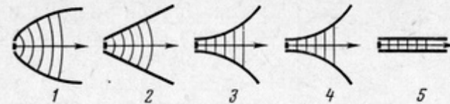
Рис. 54. Схемы рупоров различных типов:
