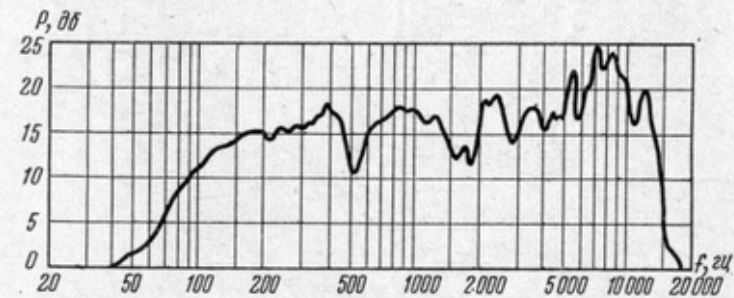
Рис. 29. Частотная характеристика громкоговорителя 25А-44
