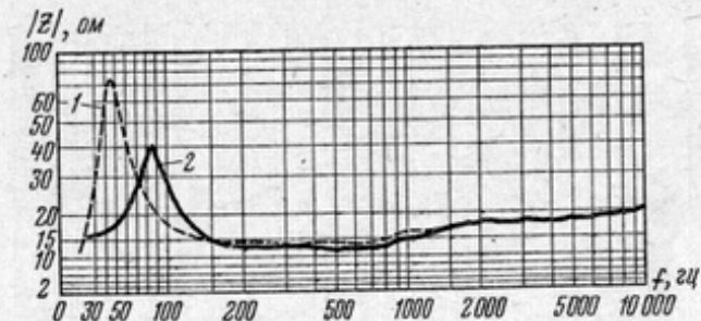
Рис. 3. Частотная характеристика модуля полного сопротивления громкоговорителя:
