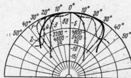
Рис. 87. Характеристики направленности:
