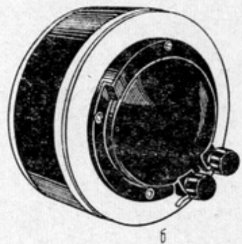
Рис. 95. Разрез (а) и общий вид (б) высокочастотной головки 1А-17:
