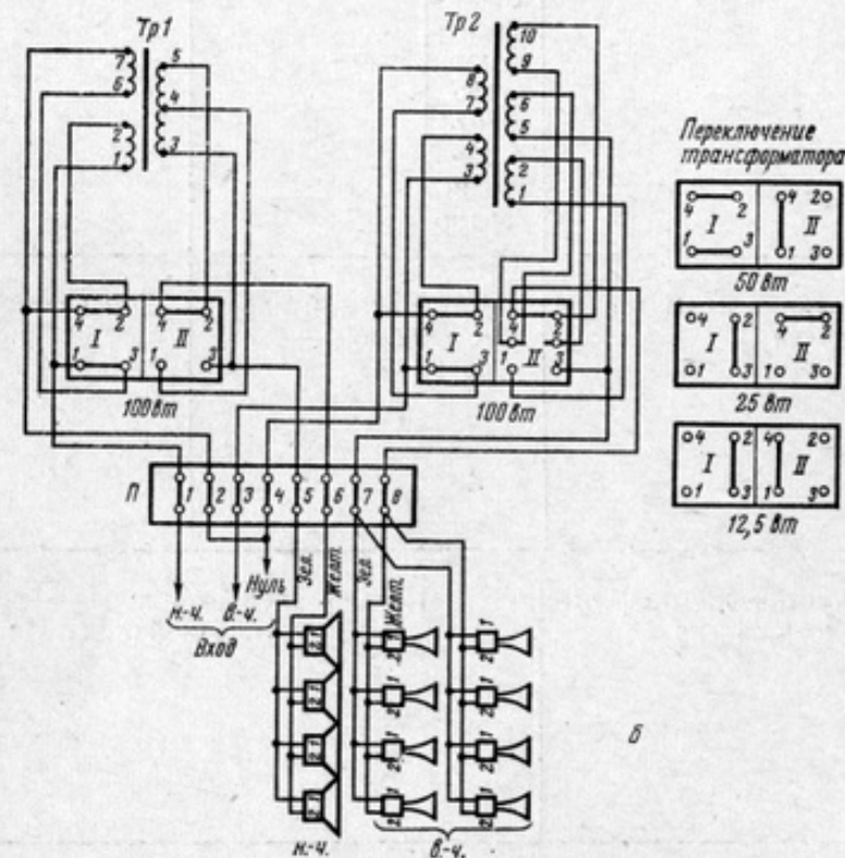
Рис. VII—7. Схема соединений громкоговорителей 30А-70(а) и 25А-24 (б)
