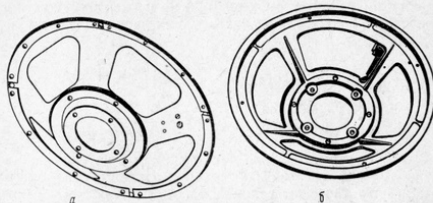
Рис. 20. Типы диффузородержателей:
