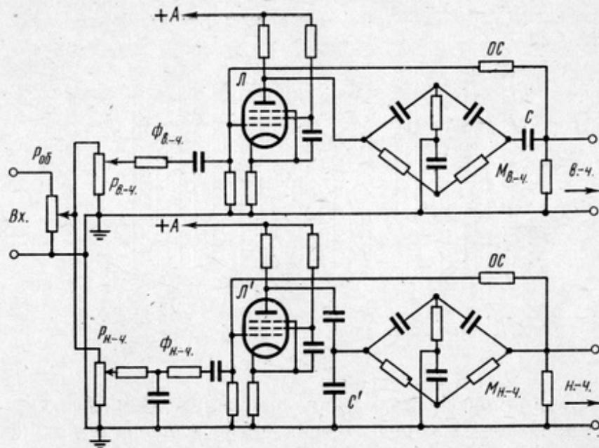
Рис. 78. Схема разделительного каскада аппаратуры КЗВТ: P_{об} ; P_{н.-ч.} ; P_{в.-ч.} — регуляторы уровня сигнала; \Phi_{н.-ч.} ; \Phi_{в.-ч.} — фильтры; ОС — цепь обратной связи; M_{н.-ч.} ; M_{в.-ч.} — балансные мосты
