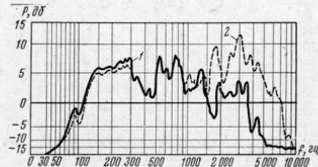
Рис. 34. Частотная характеристика головок 4А-18А в экранном ящике 25А-13:
